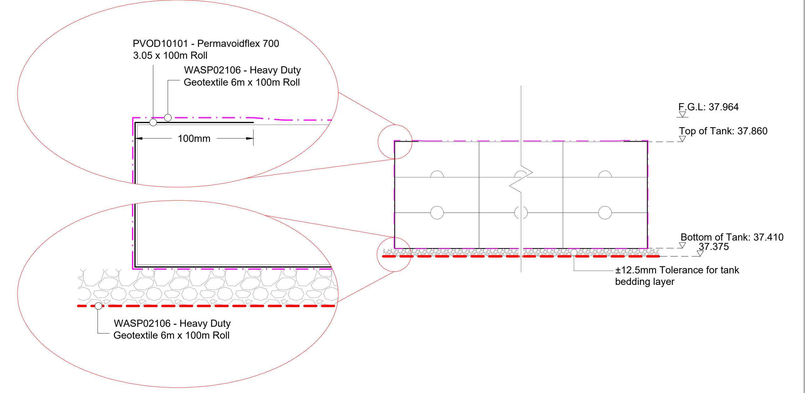
Tank Section (Scale: 1:10)
